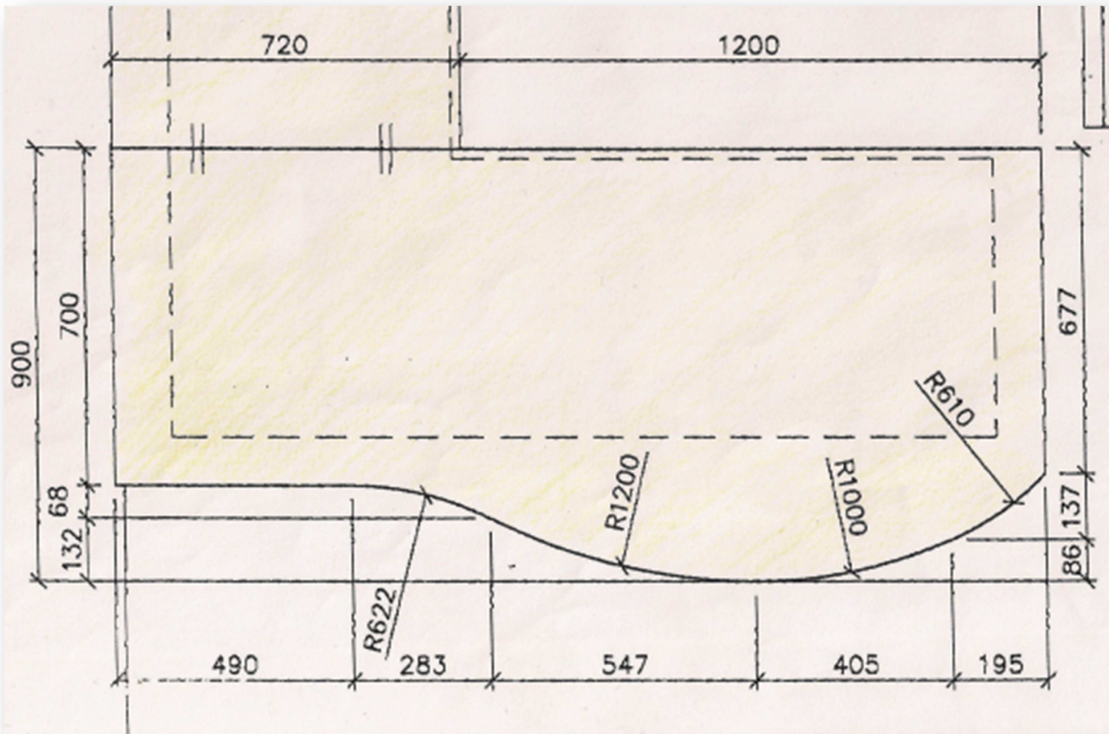
Entwurf Küchentresen-Freiform für CNC-Maschine
